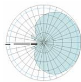
H-Plane
