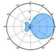
1710~2700MHz
