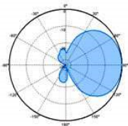
698~960MHz
