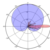
2500~2690MHz
