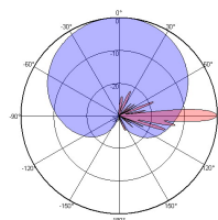
2200~2500MHz
